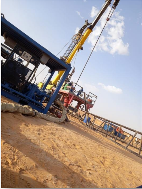
Chouech Essaida Juin 2021 Pulling Casing Kill well
